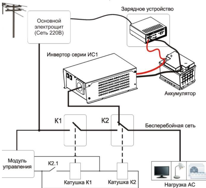
Рис.2 Схема подключения инверторов серии ИС1-У/У1/У2 к системам бесперебойного питания
