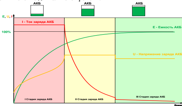
Рисунок 1 (Процесс заряда аккумуляторной батареи).
