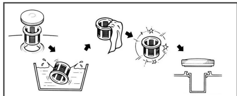
Рис.22 Чистка фильтра топливного бака
