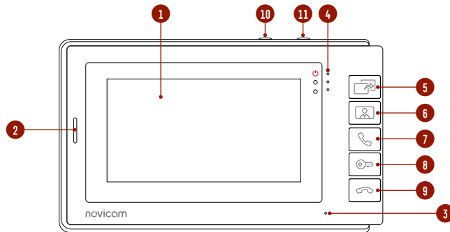
Рис. 2. Передняя панель монитора SMILE 4
