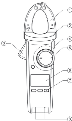
Рис. 1 Общее устройство
