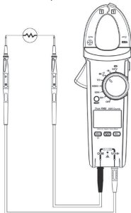
Рис. 8 Измерение сопротивления
