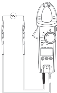
Рис. 9 Проверка целостности
