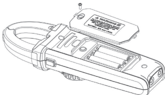
Рис. 15 Замена батареек
