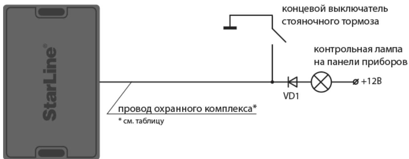
Рис. 4. Схема подключения стояночного тормоза
