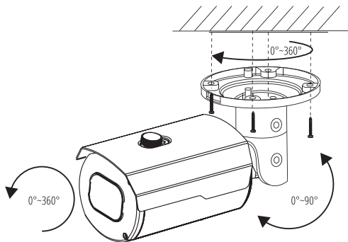
Рис. 9 Установка камеры SMART 28 | SMART 58
