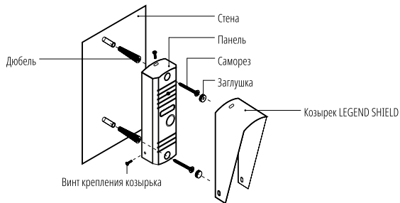
Рис. 7 Фронтальная установка вызывной панели
