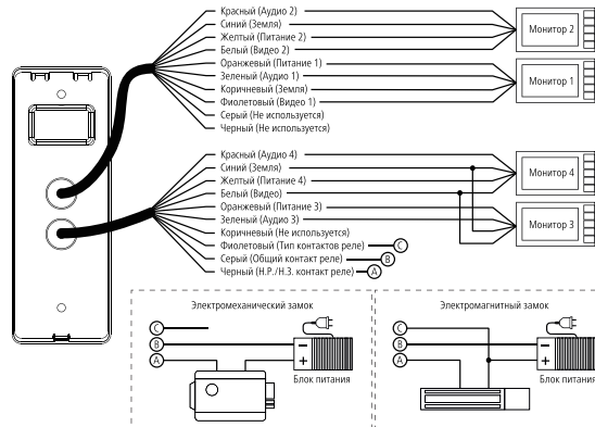
Рис. 4 Схема подключения вызывной панели FANTASY 4
