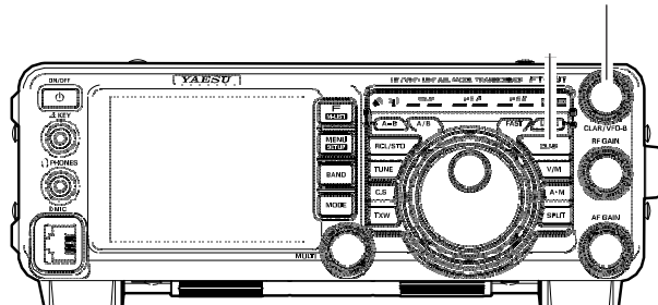
Регулятор CLAR/VFO-B Кнопка CLAR
