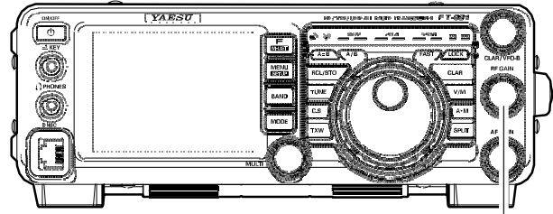
Регулятор RF GAIN
