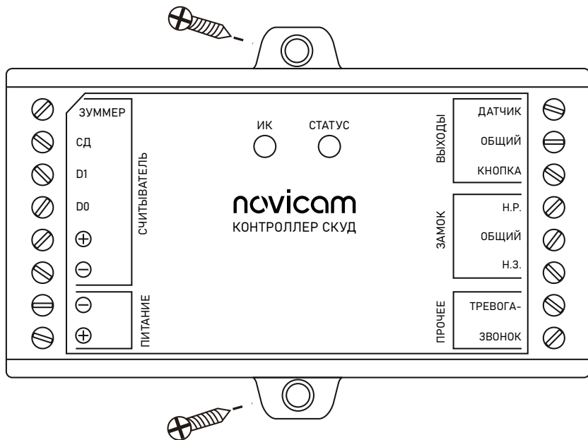
Рис. 3 Монтаж контроллера
