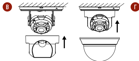
Рис. 2 Установка видеокамеры Н1Т ×0 на потолок
