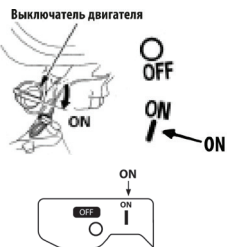
Выключатель двигателя
